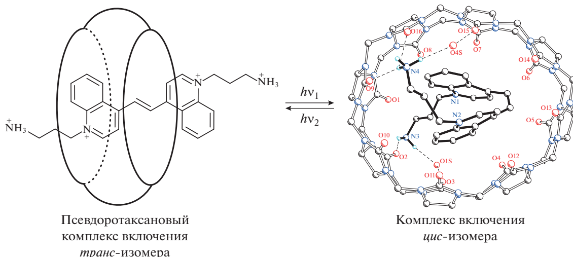
Рис. 3. Фотоуправляемая супрамолекулярная машина на основе псевдоротахсанового комплекса включения производного дихинолилэтилена с кукурбит[8]урилом.
