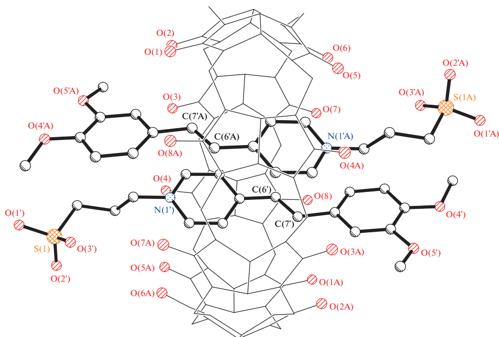
Рис. 4. Расположение двух молекул стирилового красителя в полости кукурбит[8]урила в псевдоротахсановом комплексе включения.
