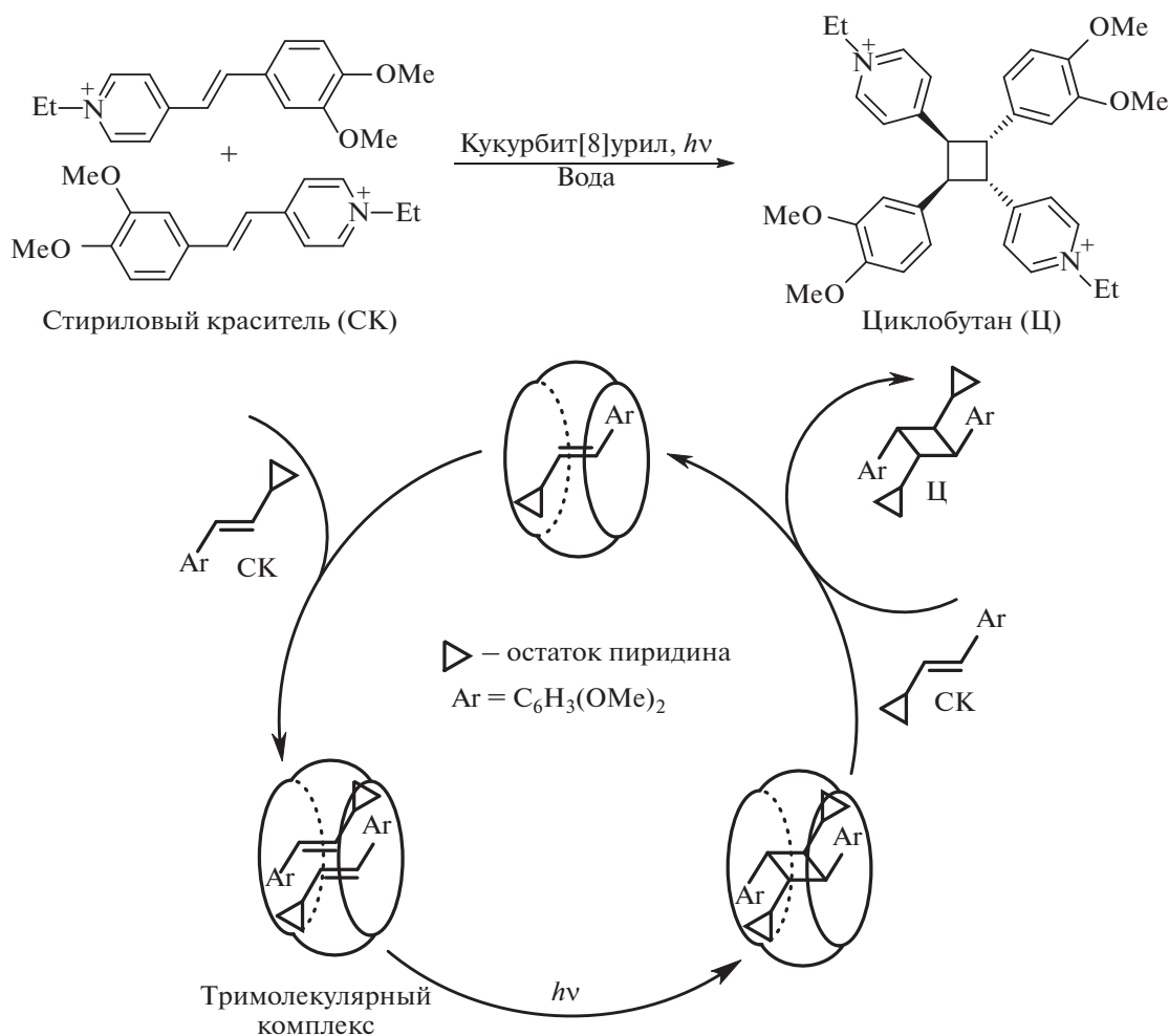
Рис. 5. Фотоуправляемый супрамолекулярный ассемблер на основе кукурбит[8]урила для сборки производных циклобутана из стириловых красителей.
